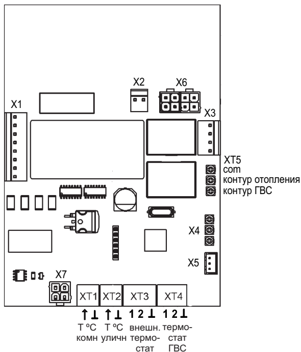
Рисунок 5. Подключение к разъёмам на плате.
