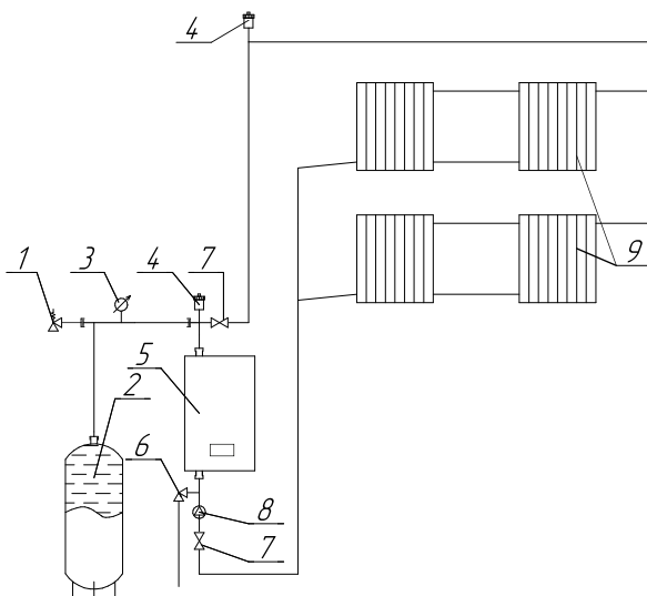
Рисунок 13. Гидравлическая схема отопительной системы
