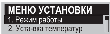
Рисунок 26. Меню установок
